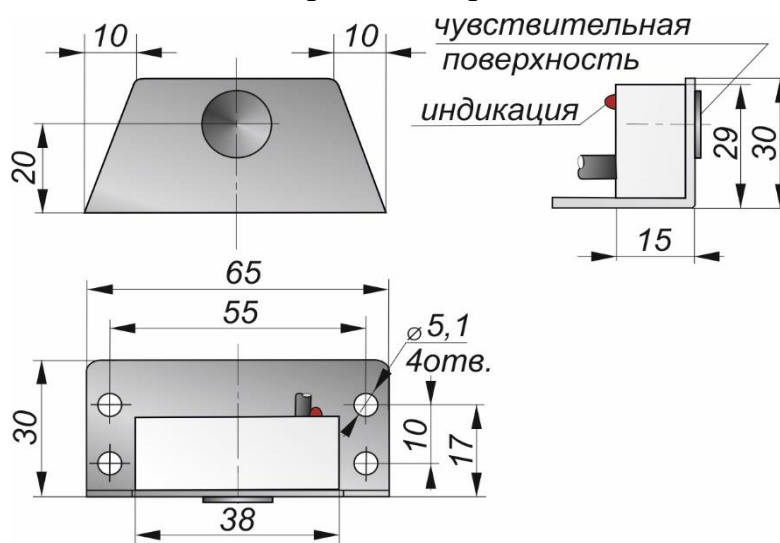
Габаритный чертеж
