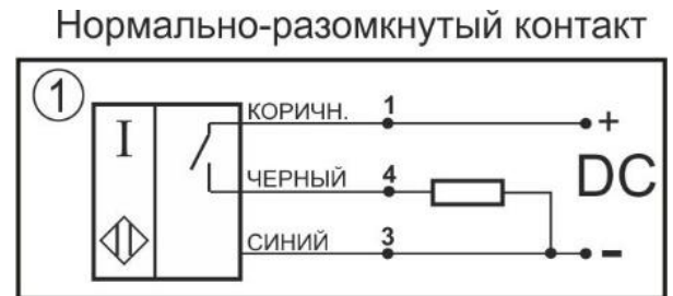
Схема соединения
