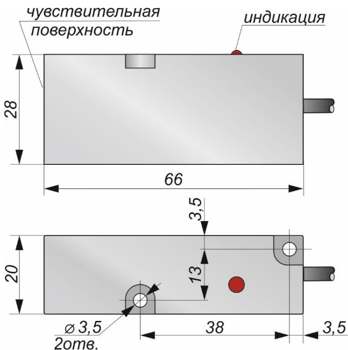
Габаритный чертеж
