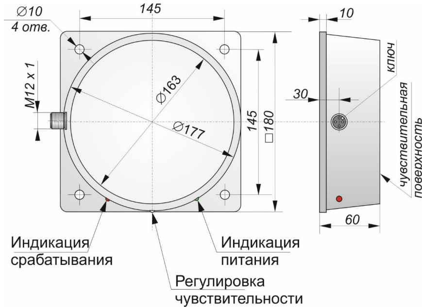
Габаритный чертеж
