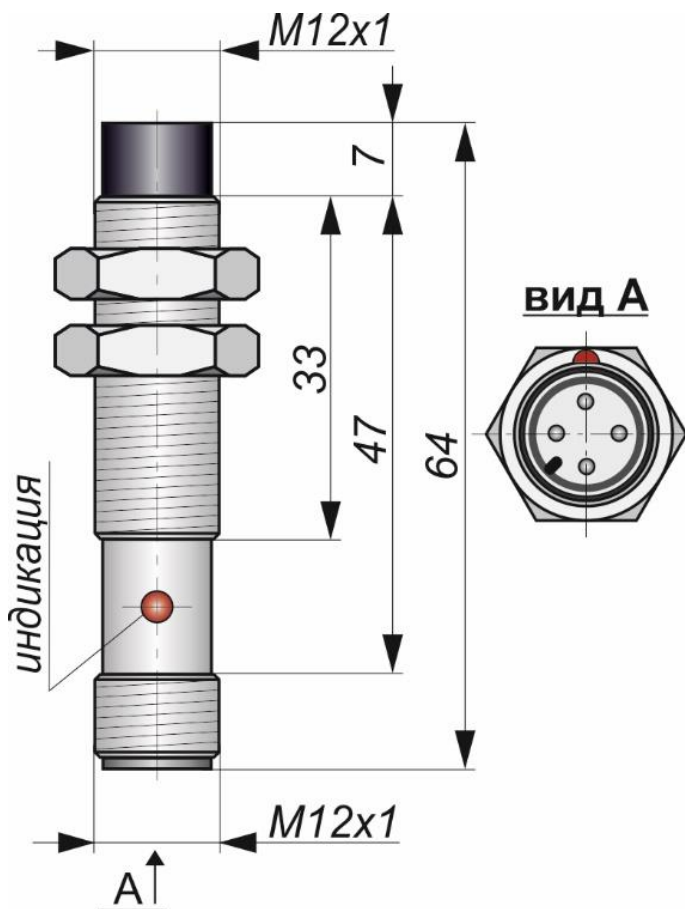
Габаритный чертеж
