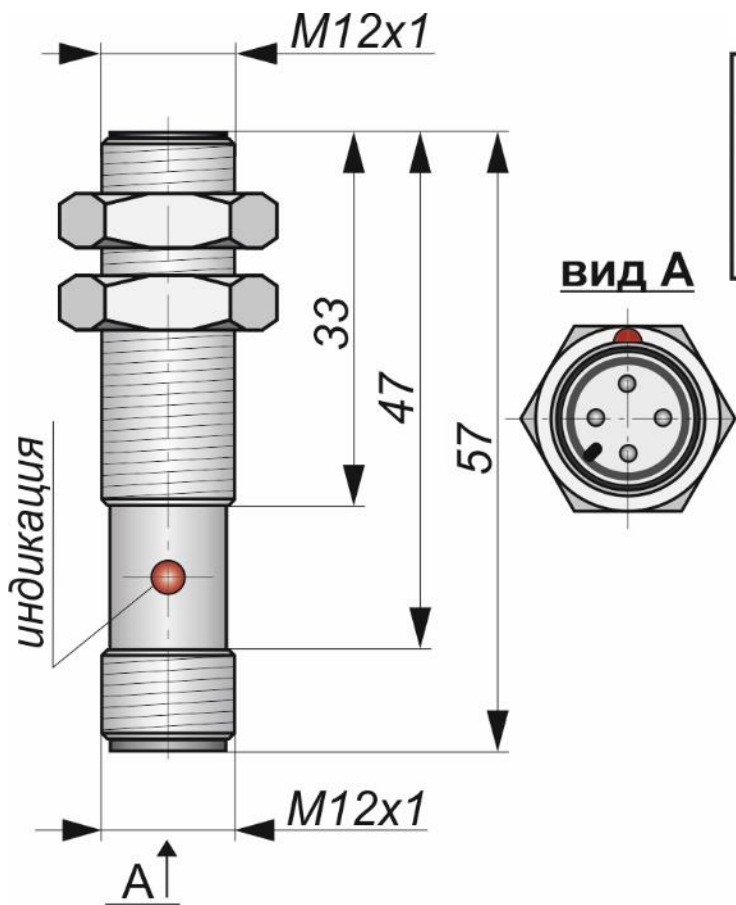
Габаритный чертеж
