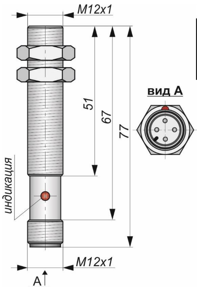
Габаритный чертеж
