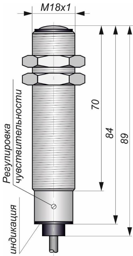
Габаритный чертеж
