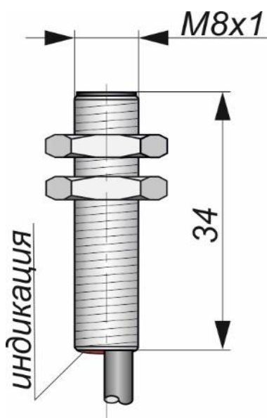
Габаритный чертеж
