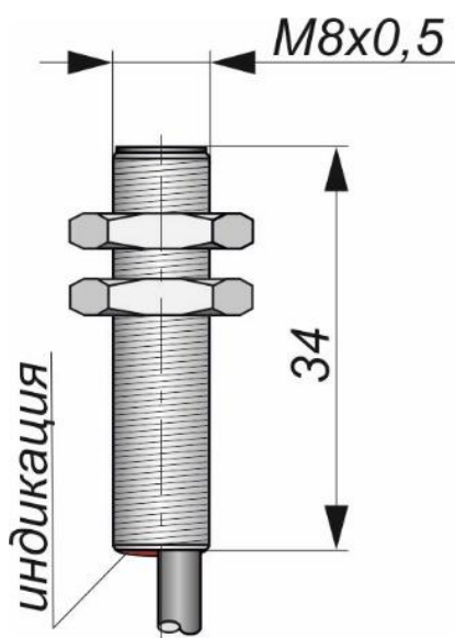
Габаритный чертеж
